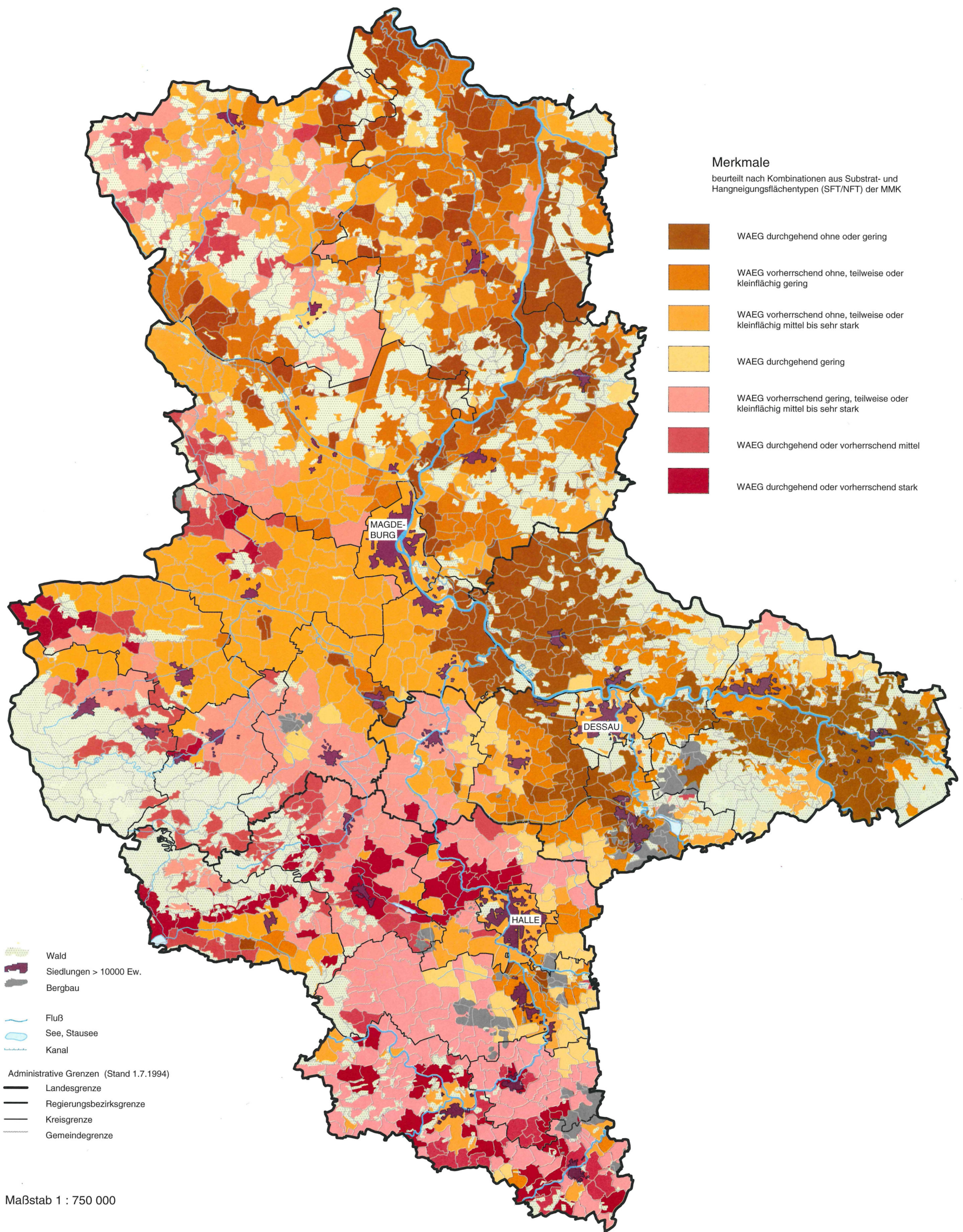
Karte 18: Gemeindebezogene potentielle Wassererosionsgefährdung (WAEG)
