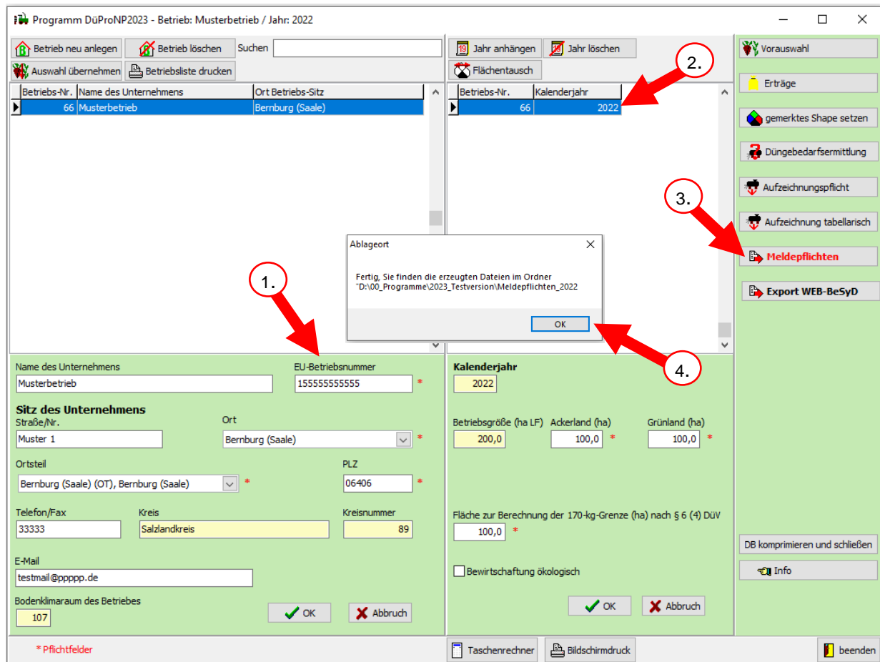
Abbildung 3: Hauptmenü
